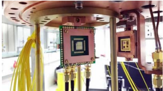
用于低温恒温器中微桥表征(一种测量薄膜力学性能的方法)的测量设置
