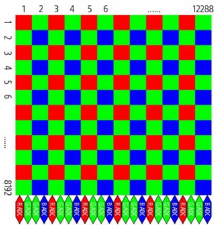
每个像素点由红绿蓝三点构成
