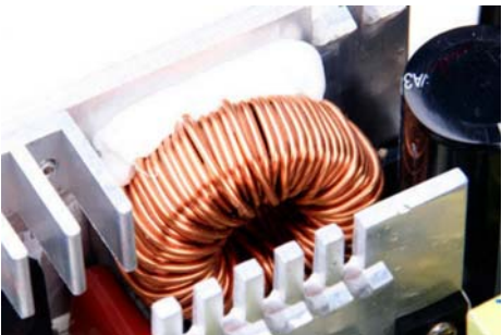
主动PFC为高端电源带来了更高的功率因数,对于电网的节能环保意义重大
