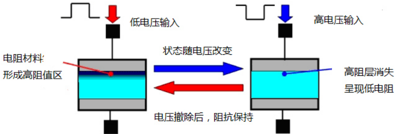
3D XPoint的可变电阻阻抗转换原理
