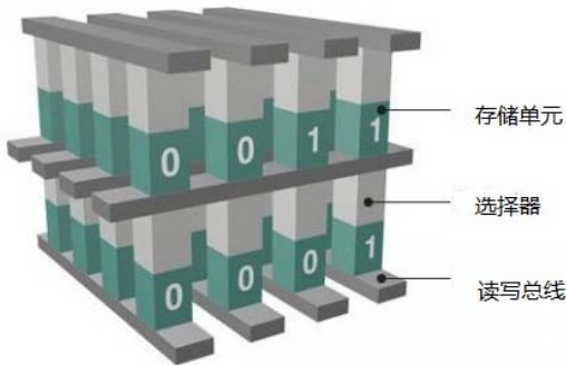
3D XPoint存储结构与原理
