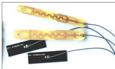
单频2.4GHz(上)与5GHz天线(下)在尺寸和结构上有较大区别
