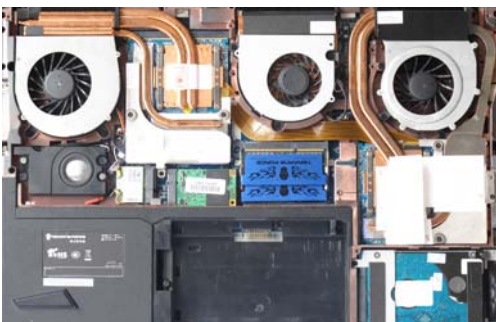
几年前的顶级游戏本大多都会采用多至3-4个风扇的散热系统,在那个时候这样的设计无可厚非
