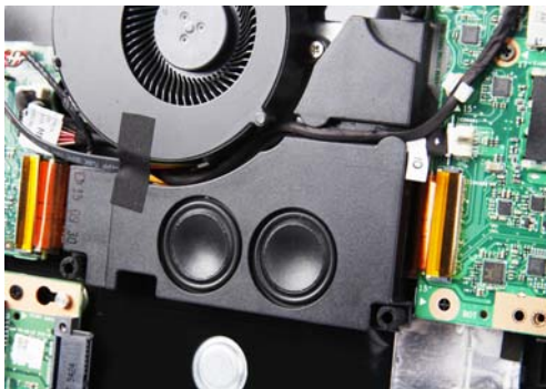
2.1声道扬声器不算少见,但像宏碁掠夺者G9-791这样每个声道都采用双单元的设计可就是头一回了,这也让该机的扬声器效果达到了惊人效果
