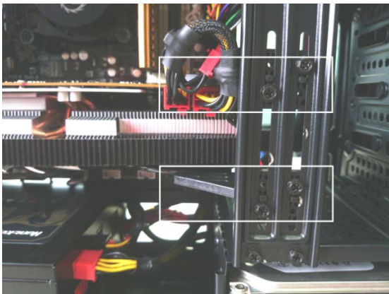
航嘉独创显卡支撑架可以将超长显卡固定得很稳当
