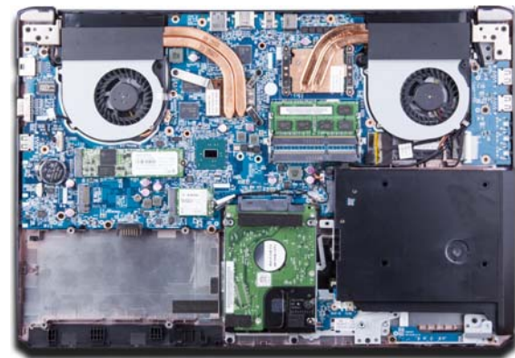
G150T 大圣本内部设计属于中规中矩的类型,各个功能模块也算是布局分明
