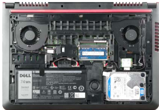
内部采用框架设计不仅能起到对元器件的保护作用，还能让走线布局更规整，有利于玩家自行维护，Inspiron 15 7000 游匣版在这方面做得非常到位
