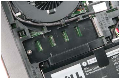
没有标配 SSD,但 Inspiron 15 7000 游匣版预留了 80mm M.2 接口,还准备了螺丝,同样很人性化
